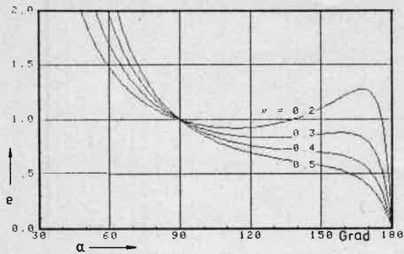
Bild 4: Empfindlichkeit e
