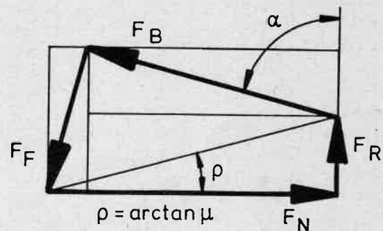
Bild 2: Kräfteplan
