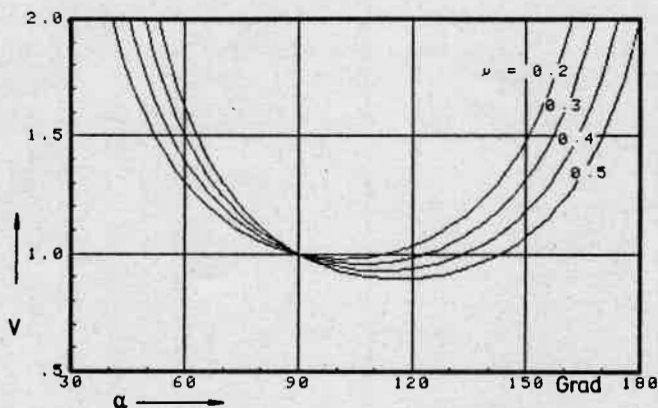
Bild 3: Verstärkungsfaktor V
