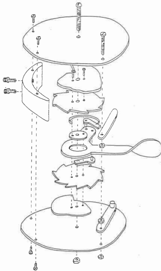
Explosionszeichnung Modell 2
