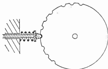
Rasterscheibe
