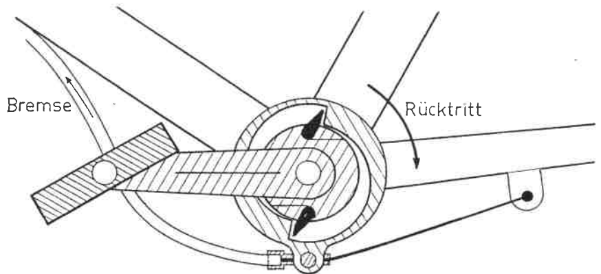
Rücktrittsgesperre im Tretlager
