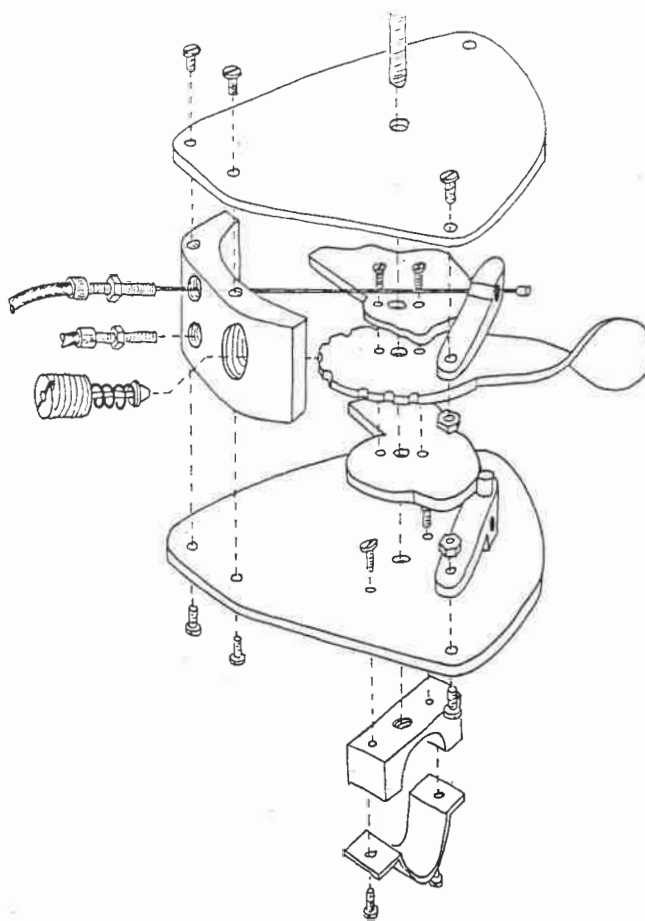
Explosionszeichnung Modell 1
