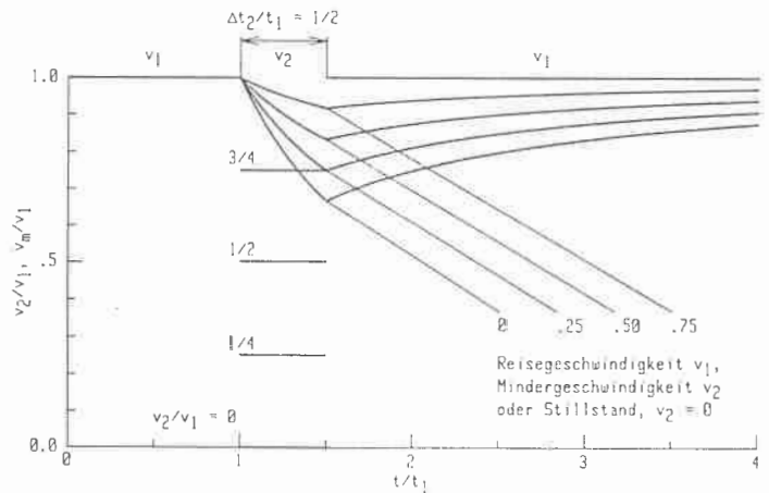
Bild 2: Radfahren wie nach Bild 1, jedoch dauert der 'Hindernis'-Zustand die Hälfte des ersten Fahrzeugzustandes
