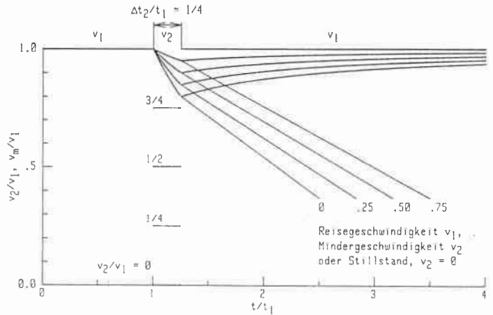
Bild 1: Radfahren mit 'Hindernissen', mittlere Geschwindigkeit. 'Hindernis'-Zustand dauert ein Viertel des ersten Fahrzeugzustandes mit der gewählten Reisegeschwindigkeit
