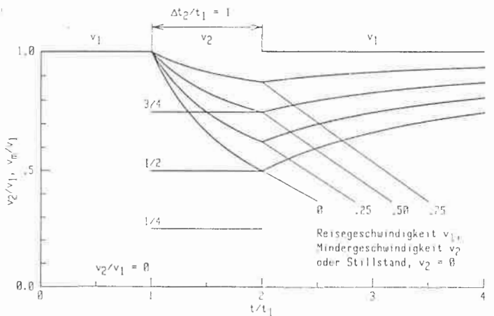
Bild 3: Radfahren wie nach Bild 1, jedoch dauert der 'Hindernis'-Zustand so lange wie der erste Fahrzeugzustand
