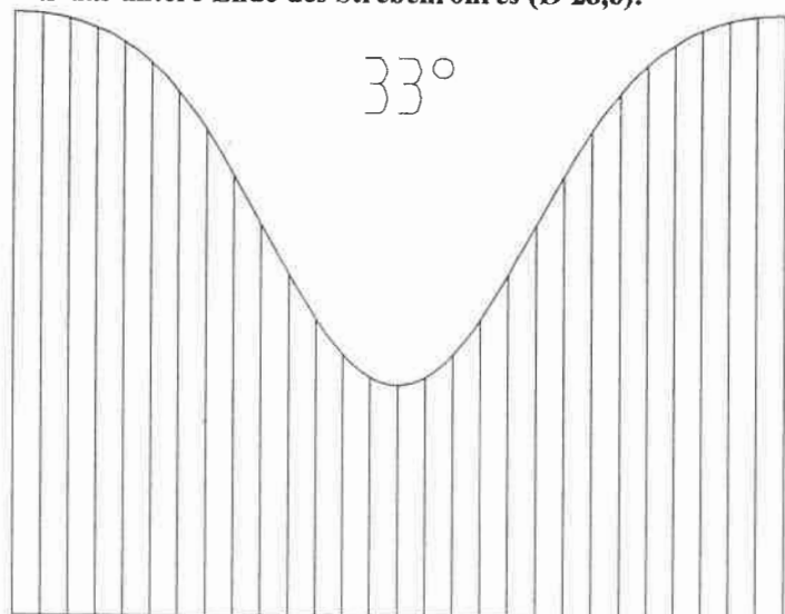
Für das untere Ende des Strebenrohres (Ø 28,6):
